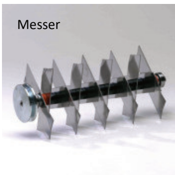
Doppelmesserschneidesystem
